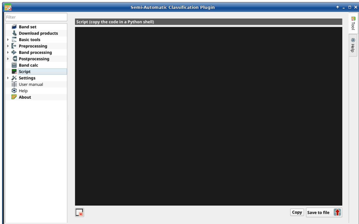
Abb. 46: Script
