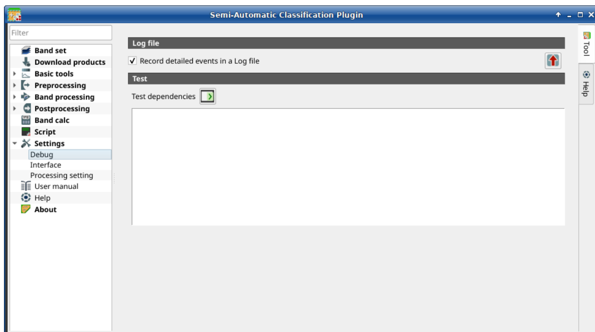
Abb. 1: Debug
