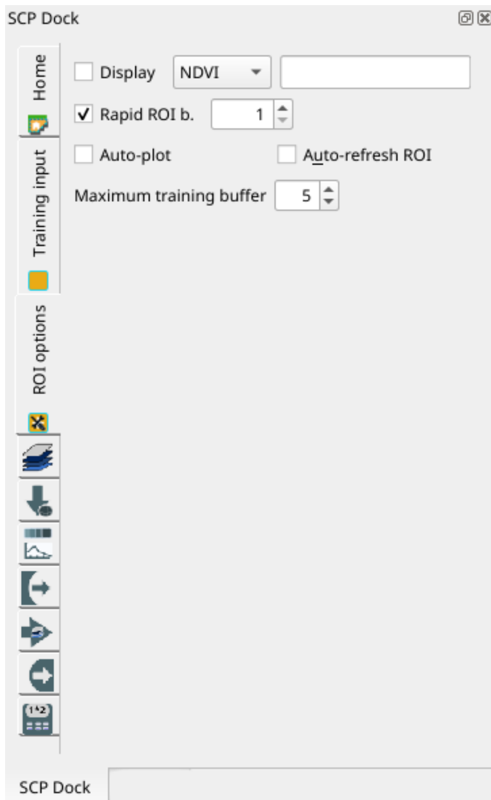
Abb. 7: ROI options
