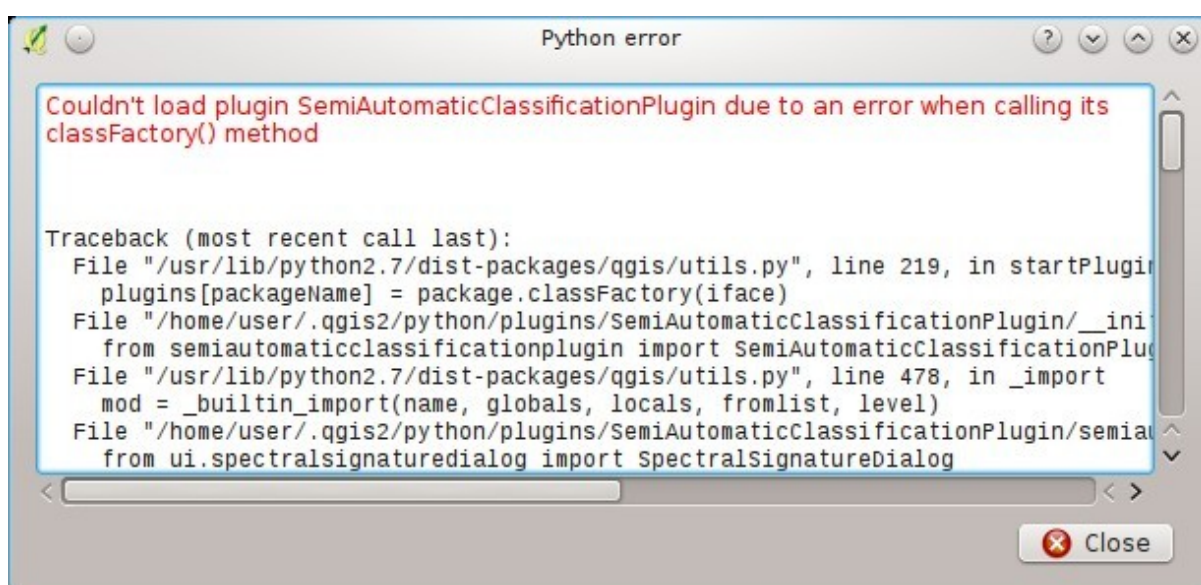
Abb. 2: Error message
