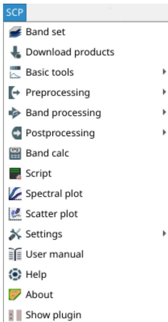
Abb. 1: SCP menu
