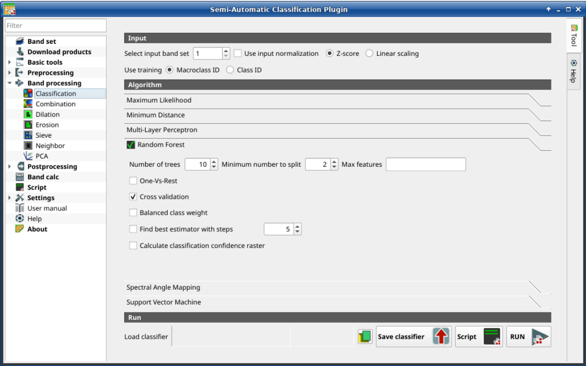
Abb. 31: Random Forest
