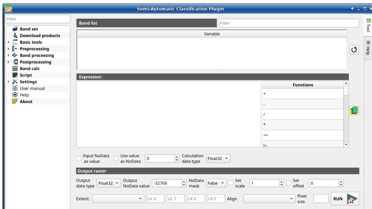
Abb. 45: Band calc
