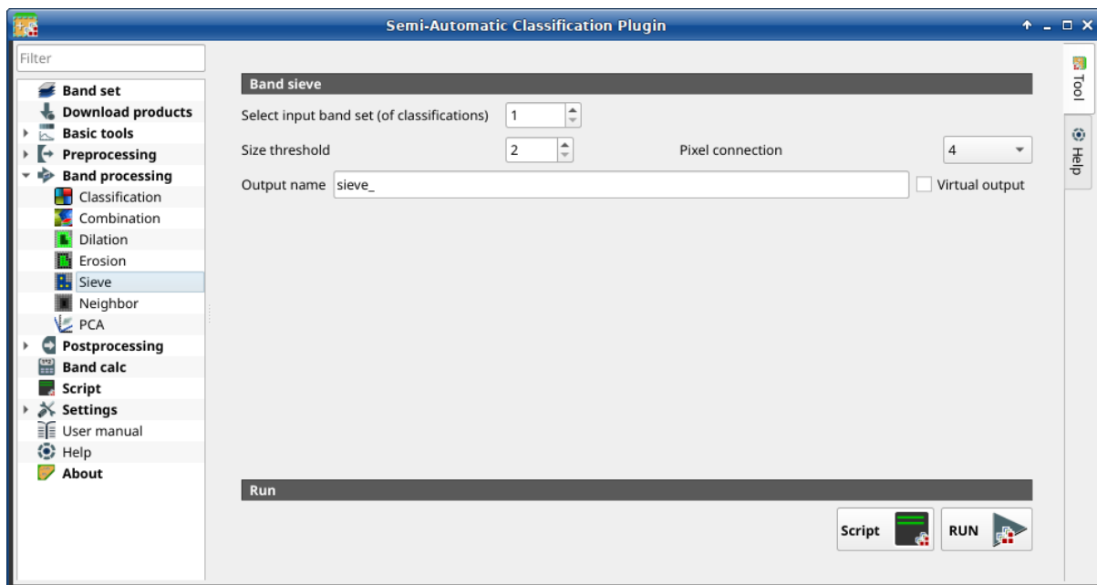
Abb. 37: Sieve
