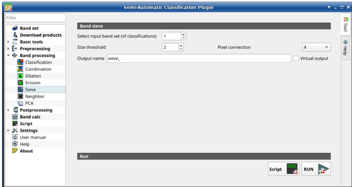
Gambar. 37: Sieve
