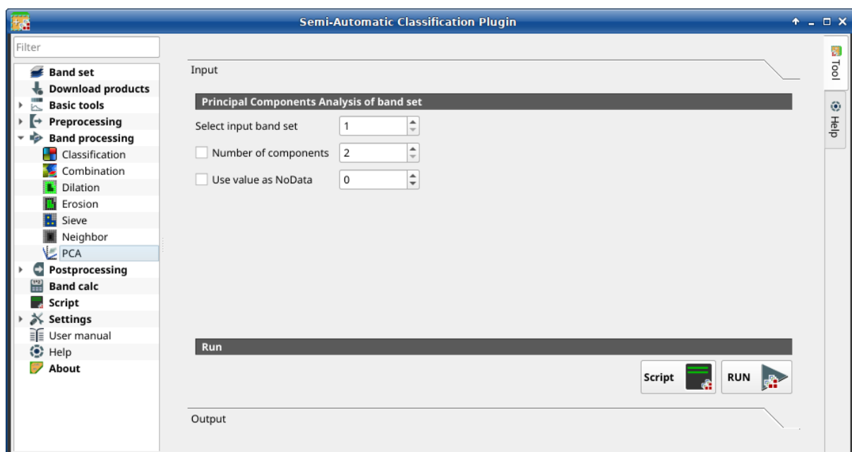
Gambar. 39: PCA
