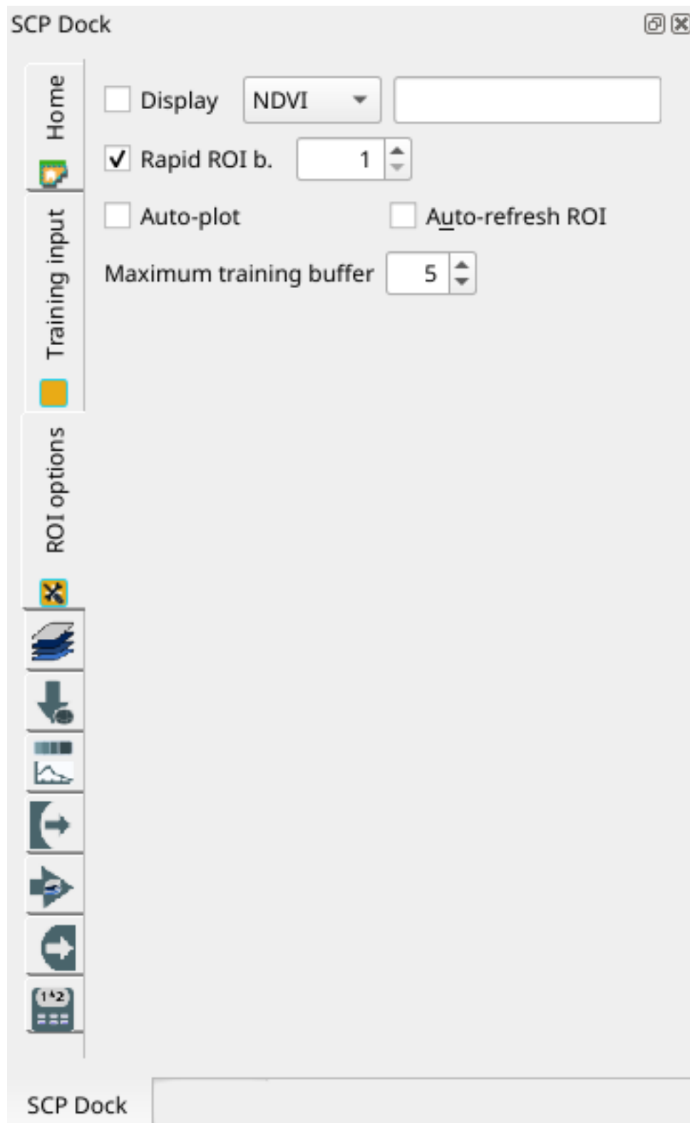
Gambar. 7: ROI options
